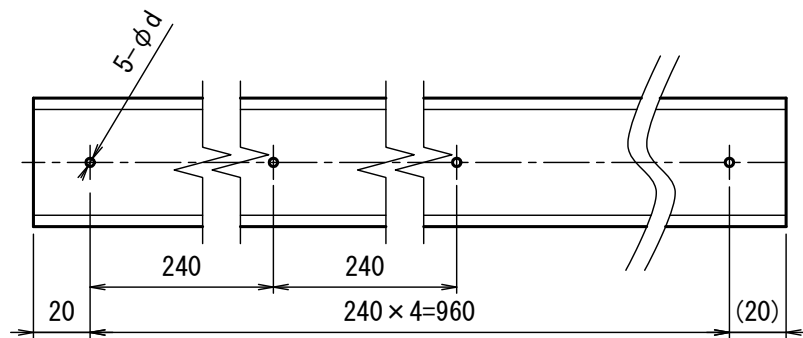
製品裏面釘穴図
